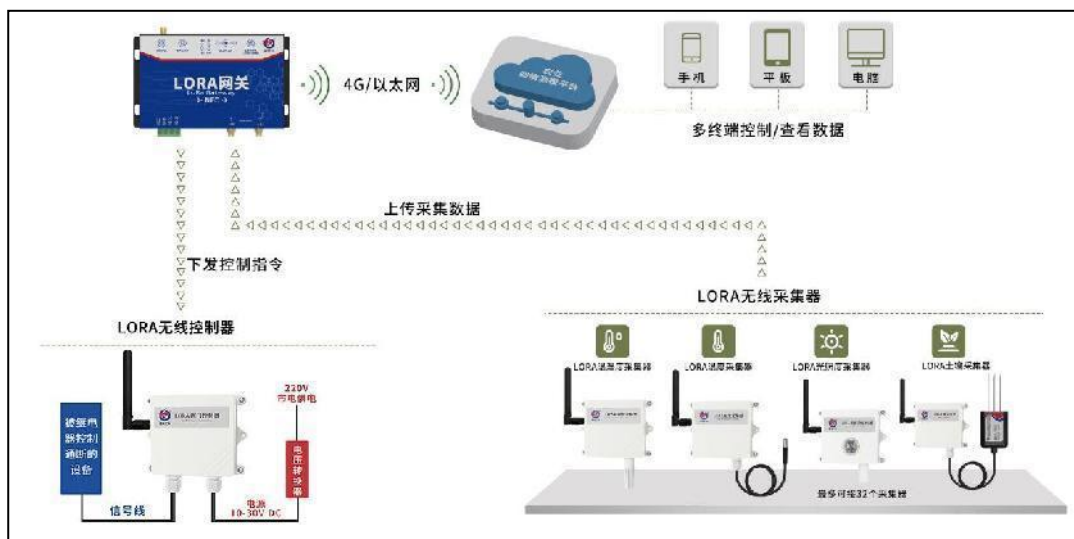
网络型 LORA 网关使用拓扑图
