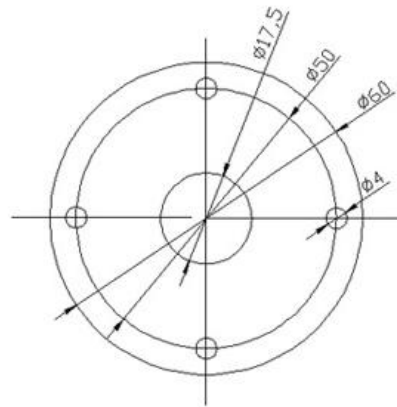
② 用螺丝将法兰盘固定在非风管上
