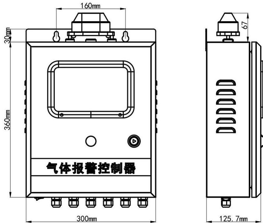
控制器尺寸 (单位 mm)
