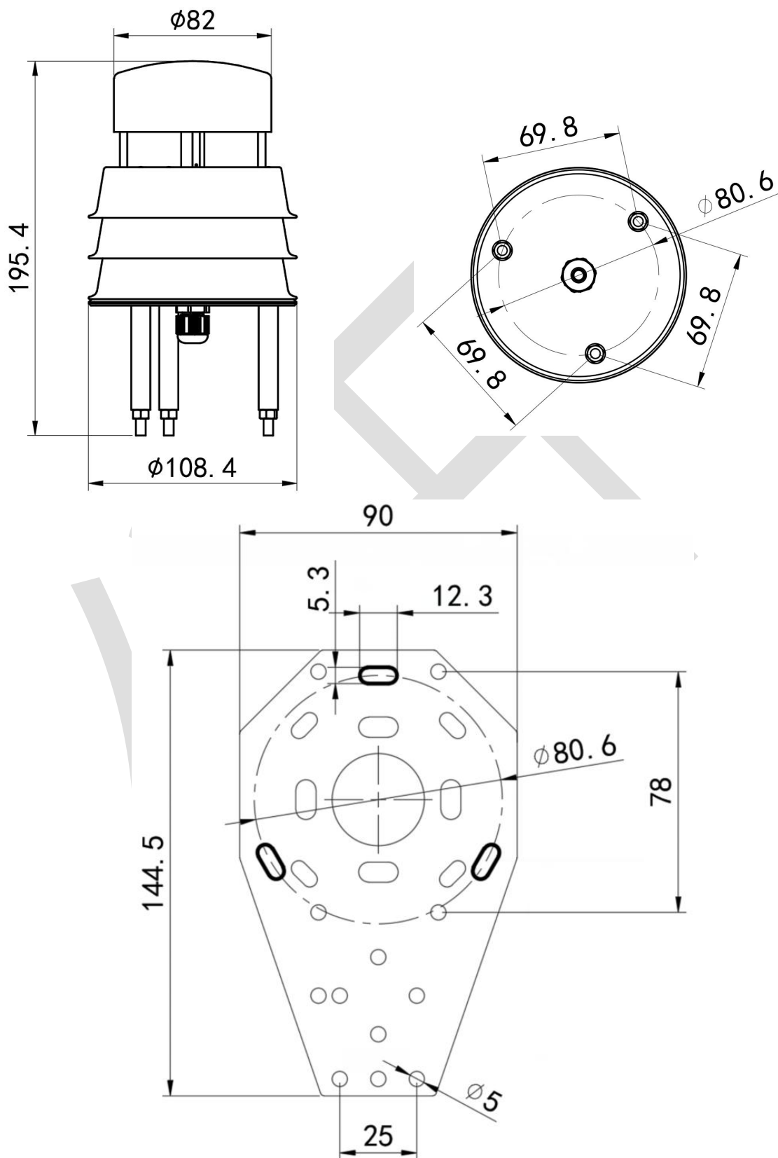
设备尺寸图（单位 mm）
