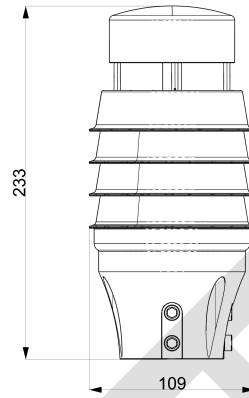
设备尺寸图（单位 mm）
