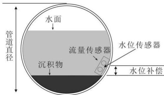
有沉积物管道的安装位置
