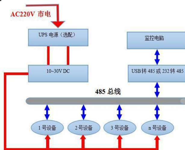
系统方案图
