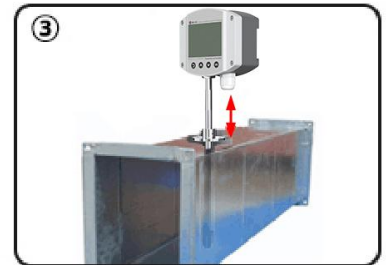
③ 将设备插入到法兰盘中，完成安装
